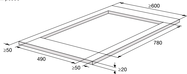
Installation posée
