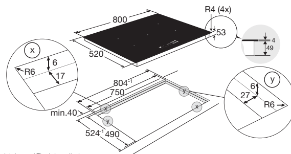
Vlak inbouw / Flush installation
